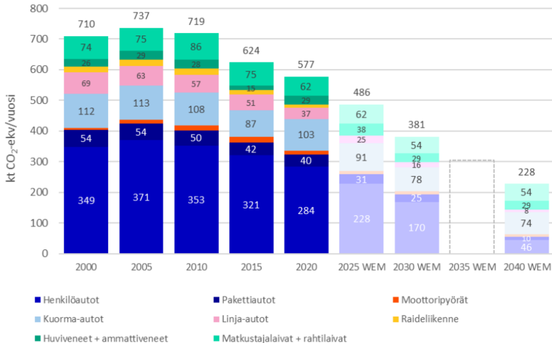
Liikenteen päästöt Helsingissä kulkumuodoittain, 1000 tonnia CO 2 -ekv / vuosi
